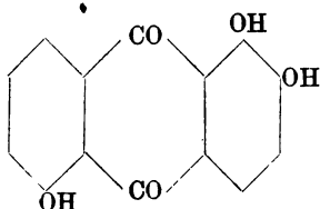
Oxyanthrarufin 1 : 2 : 5.
